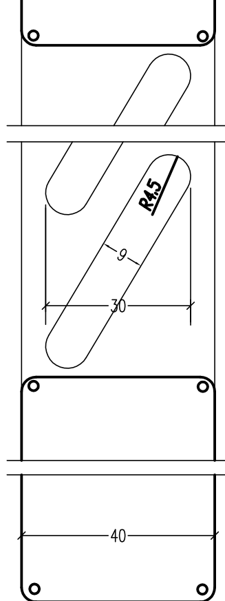
Sección 8
