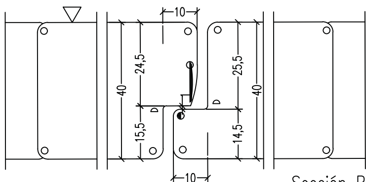
Sección B-B
