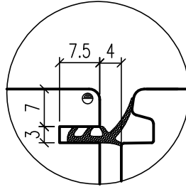
Variante 1 Goma en el cierre central On-Off
