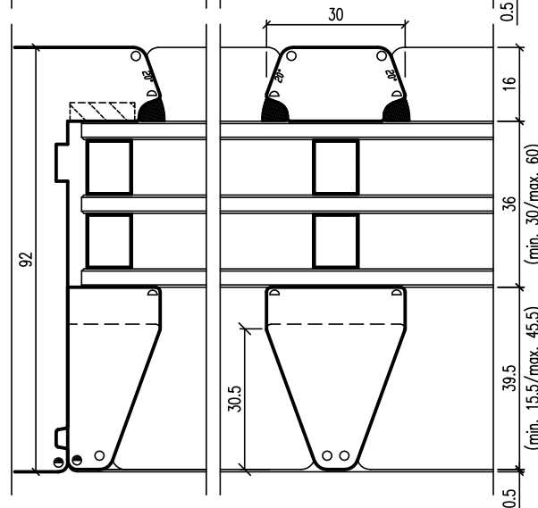
VARIANTE 1 LARGUEROS Y TRAVESAÑOS A 20°
