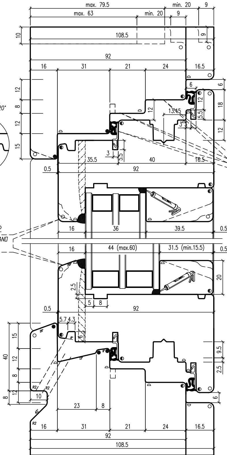
Variante 3 Goma acustica On-Off
