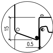
Variante 1 Interior marco a 20°
