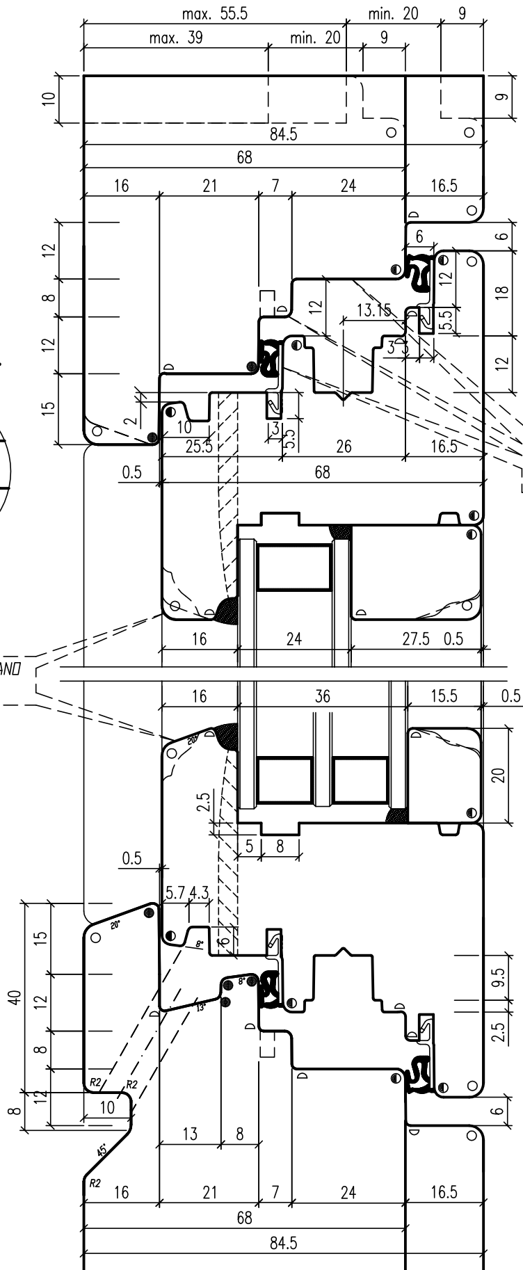
Variante 1 Interior marco a 20°
