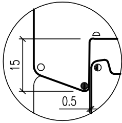
Variante 1 Interior marco a 20°
